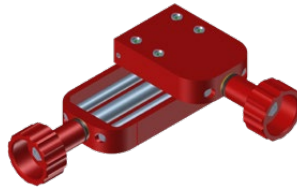
ZSP-0466-46-00-00-1 Erweiterter Kreuzschlitten 0-76 mm auf und ab 0-35 mm links-rechts
