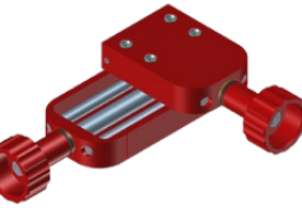
ZSP-0466-46-00-00-1 Erweiterter Kreuzschlitten 0-76 mm auf und ab 0-35 mm links-rechts
