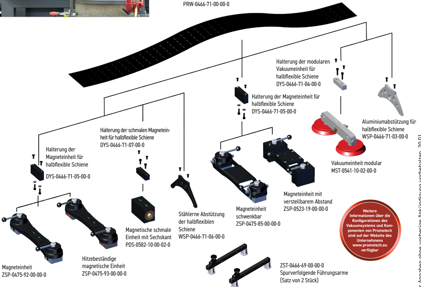
Laznge flexible Schiene 1,88 m Minimaler Krümmungsradius von 1,25 m PRW-0466-71-00-00-0
