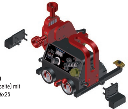
BLO-0466-47-01-00-0 Magnetblöcke (vorne) mit erhöhter Leistung M5x25
