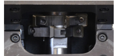
2 Dreh-Fräsköpfe mit je fünf 4-seitigen Wendeschneidplatten
